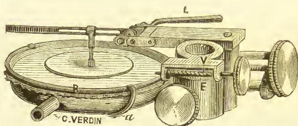
Fig. 2. — Tambour enregistreur.
